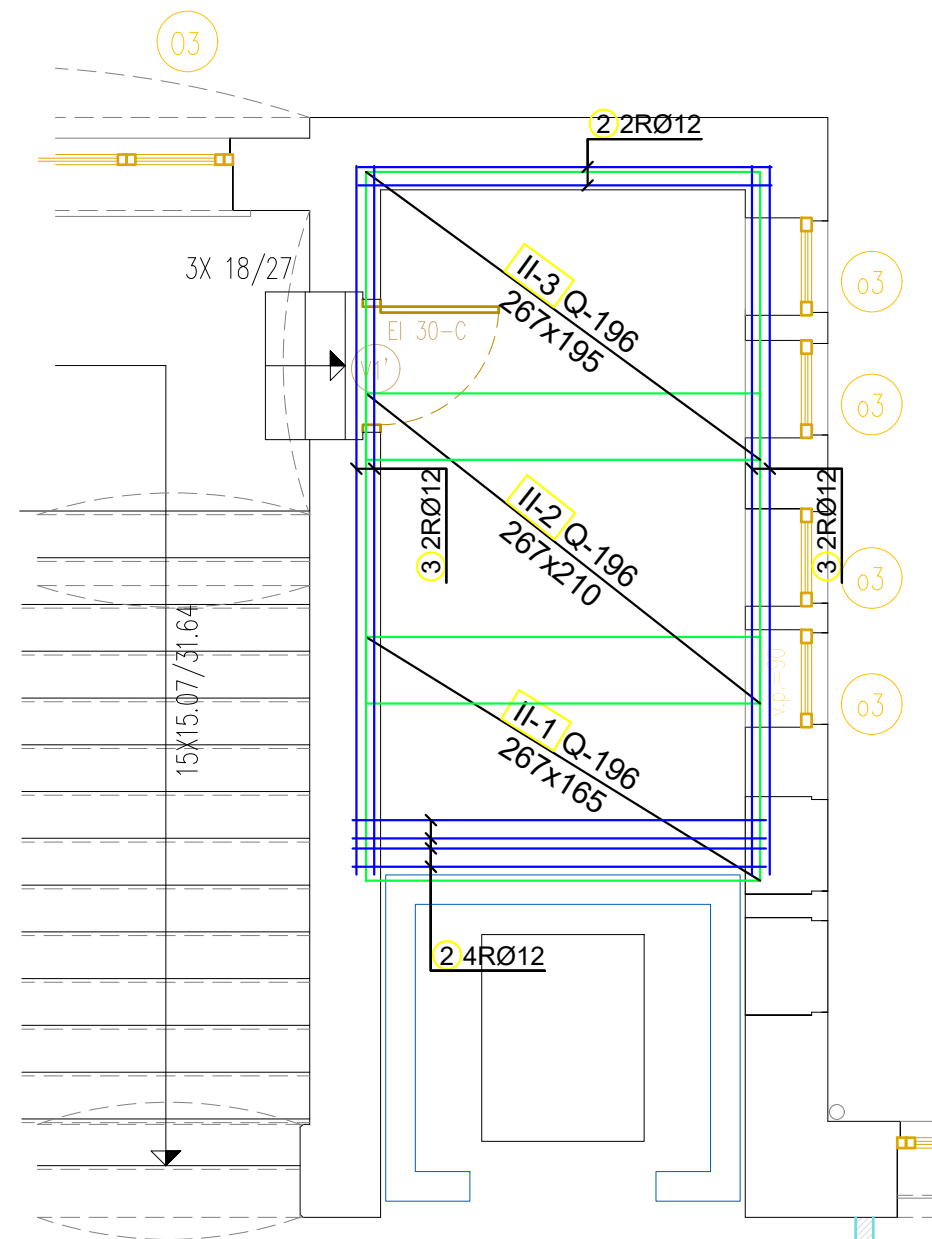
armatura ZGORAJ
