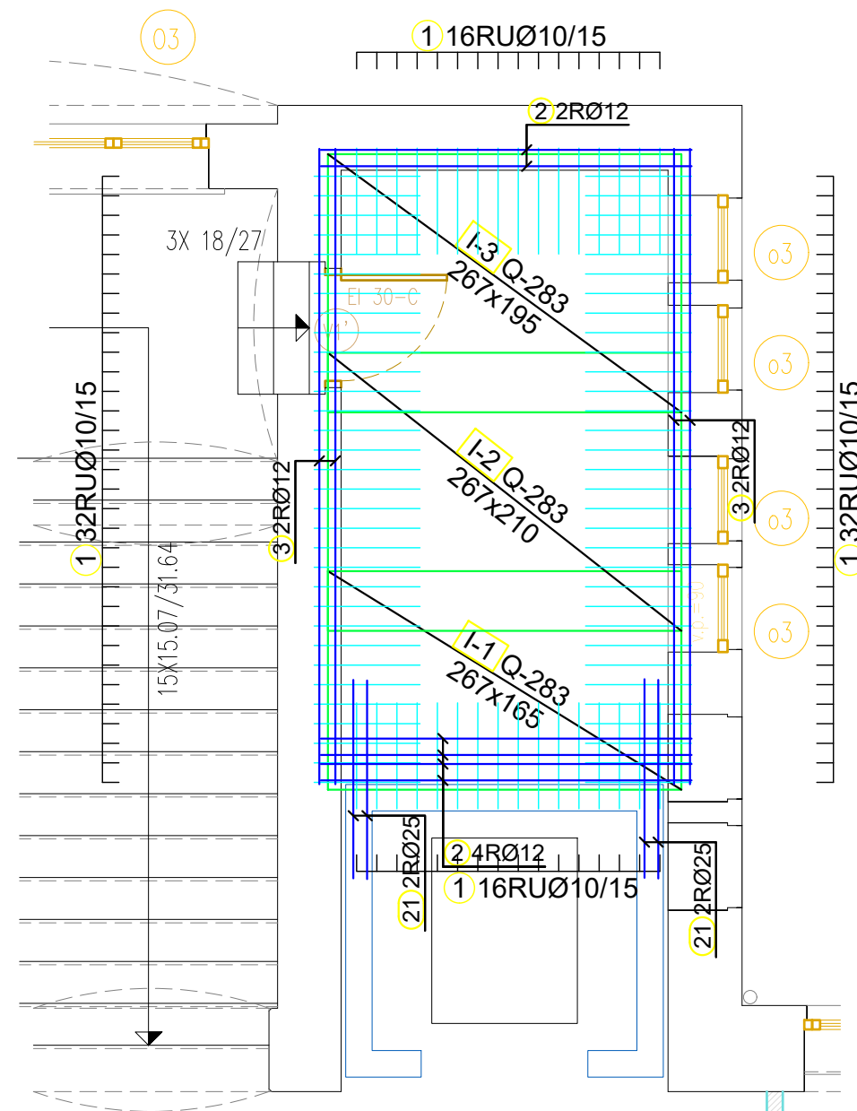
armatura SPODAJ
